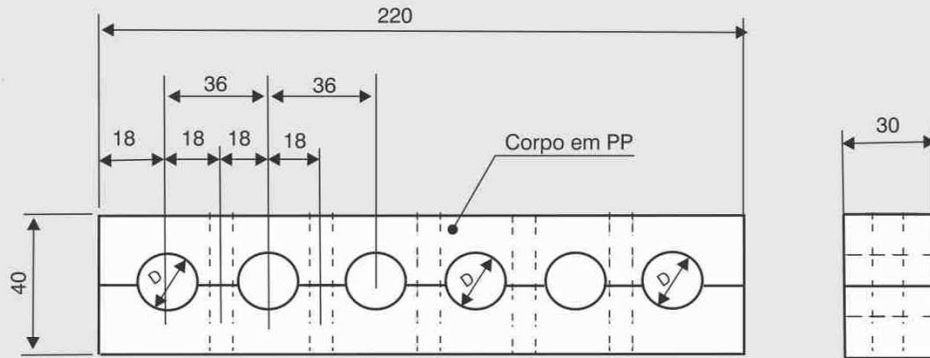
BRAÇADEIRA PARA 6 TUBOS: Diâmetros 22 e 25 mm.
