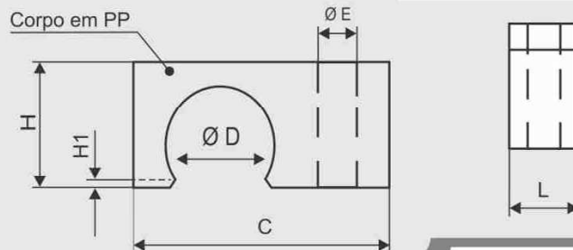
BRAÇADEIRA PARA 1 TUBO: Diâmetros 15 / 16 / 20 / 22 e 25 mm.
