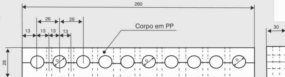
BRAÇADEIRA PARA 10 TUBOS: Diâmetros 9,5 / 12,7 e 15 mm.
